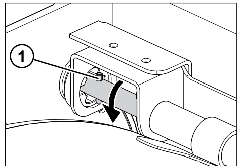
Fig. 6-10: Rotazione della manovella per allungamento posteriore
