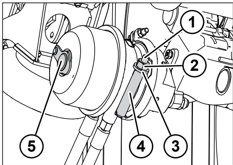
Fig. 5-13: Accumulatore a molla con dispositivo di rilascio di emergenza
