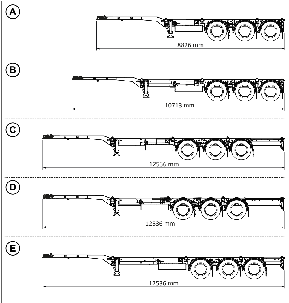
Fig. 12-1: Vista generale Dimensioni rimorchio
