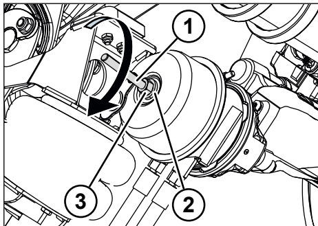
Fig. 5-14: Attivare la vite per il rilascio d'emergenza
