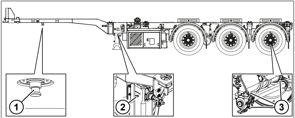
Fig. 9-1: Punti di lubrificazione Box Liner TU70
