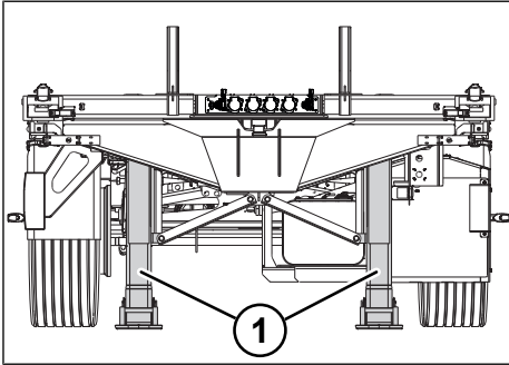
Fig. 5-2: Martinetti di supporto estratti 1 Martinetti di supporto
