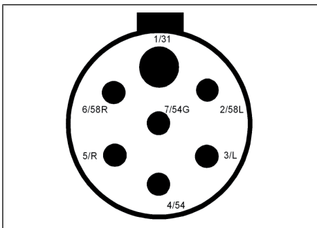
Fig. 12-4: Presa ISO N 1185, 7 poli
