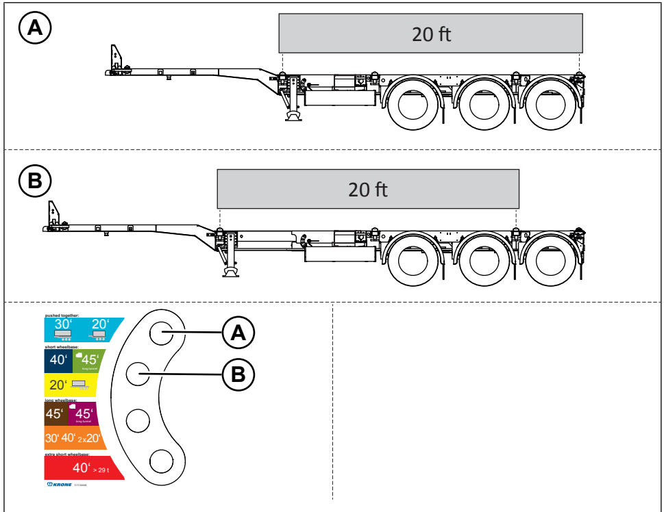
Fig. 6-27: Vista generale delle posizioni dei container
