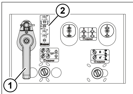
Fig. 5-16: Leva di azionamento delle sospensioni pneumatiche
