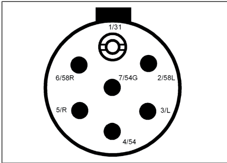
Fig. 12-3: Presa ISO S 3731, 7 poli
