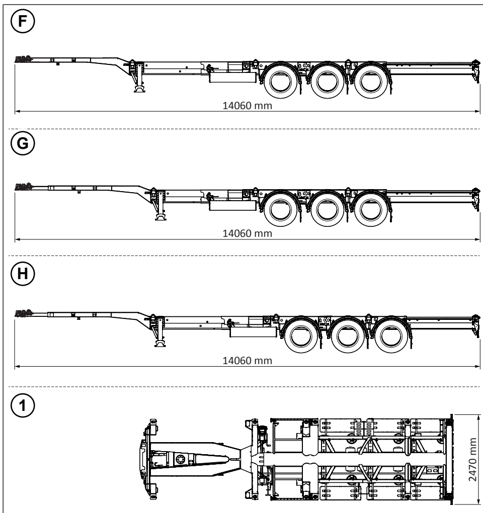
Fig. 12-2: Vista generale Dimensioni rimorchio
