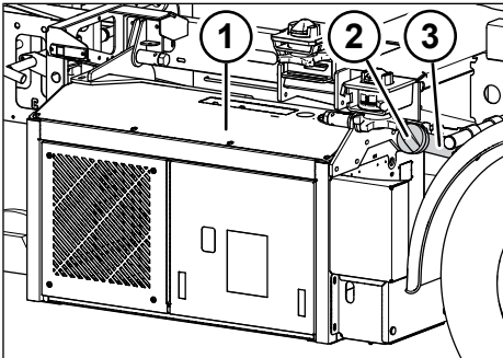
Fig. 6-32: Rifornimento del gruppo elettrogeno
