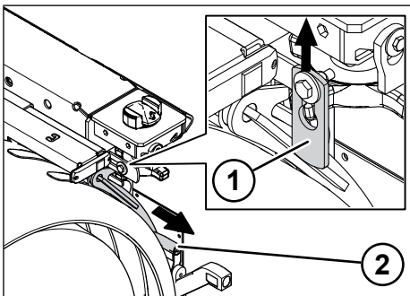
Fig. 6-3: Sbloccaggio della manovella per allungamento posteriore
