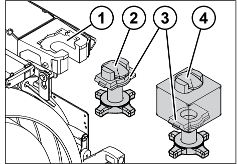
Fig. 6-24: Sostituzione del bloccaggio
