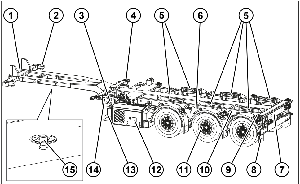
Fig. 3-1: Vista generale Box Liner TU70
