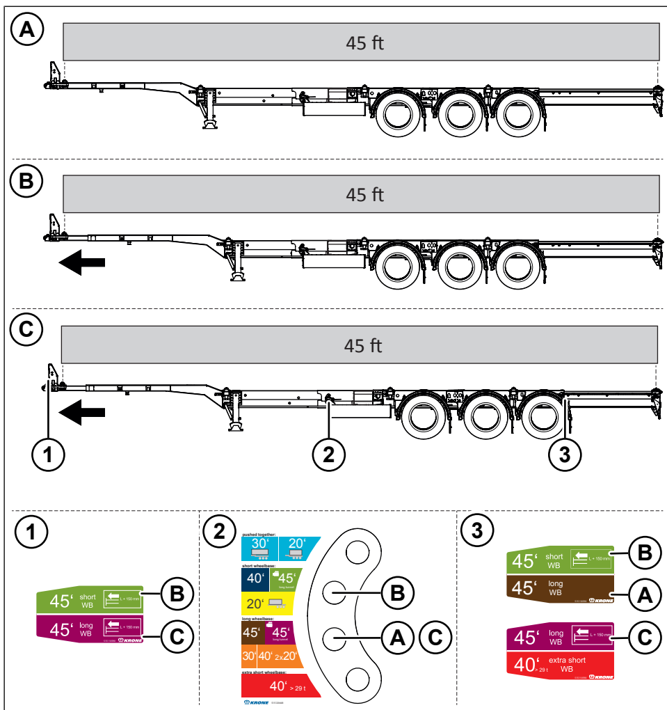
Fig. 6-30: Vista generale delle posizioni dei container
