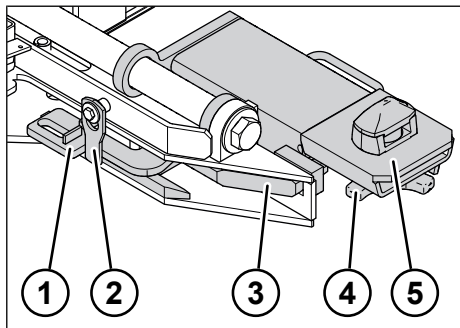
Fig. 6-16: Meccanismo di presa container in posizione di presa
