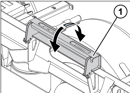
Fig. 6-23: Appoggio intermedio ribaltabile
