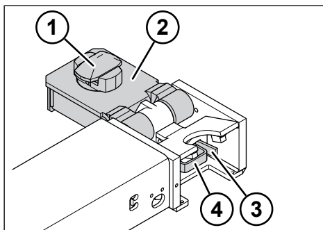
Fig. 6-20: Meccanismo di presa container in posizione di presa
