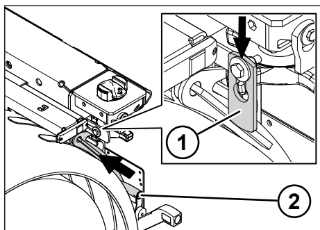
Fig. 6-8: Fissaggio della manovella per allungamento posteriore
