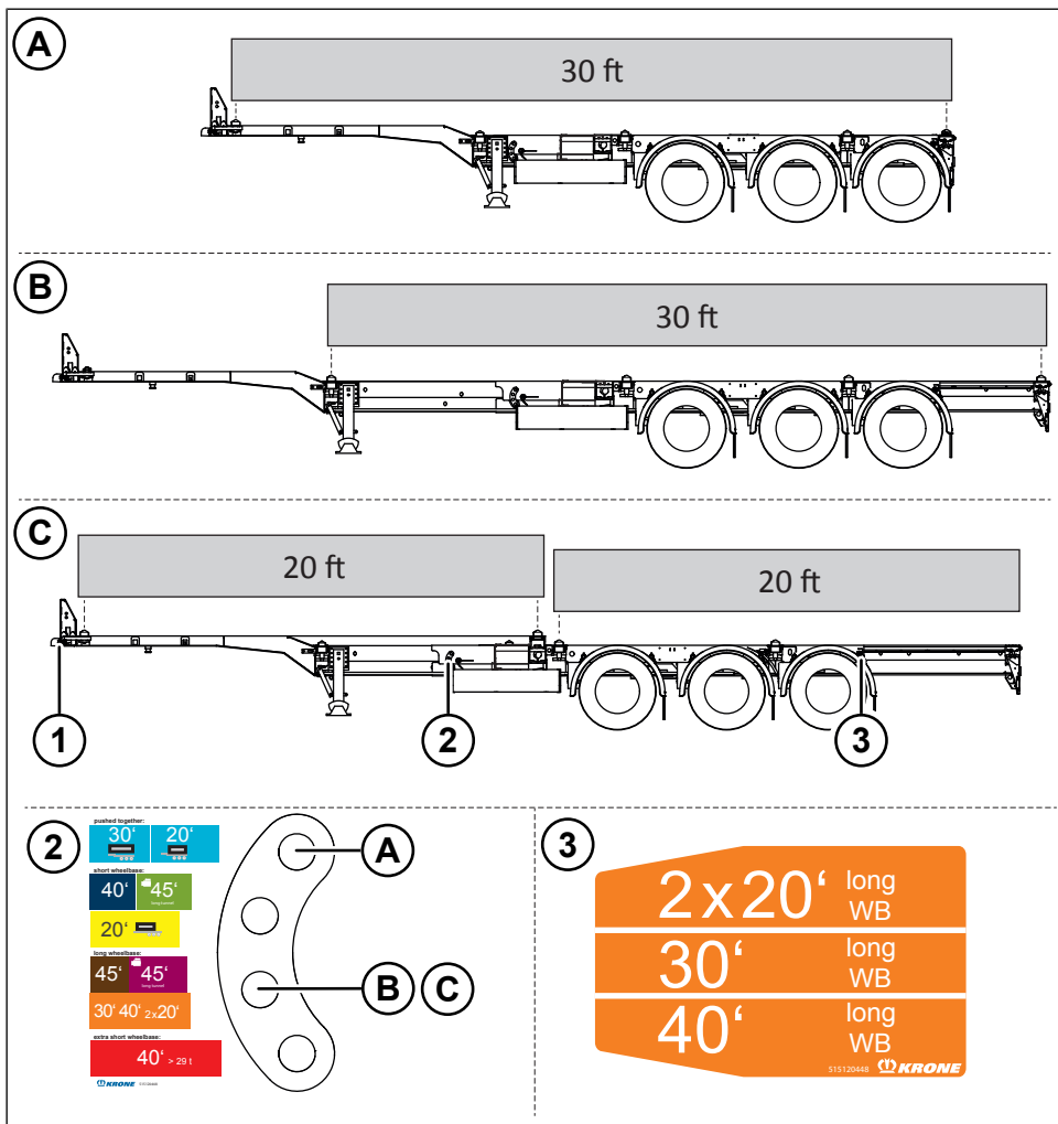
Fig. 6-28: Vista generale delle posizioni dei container
