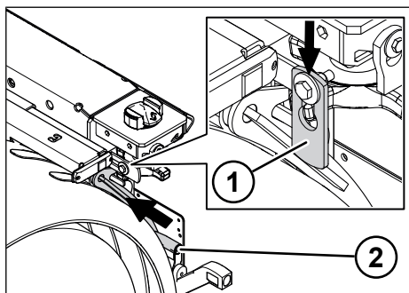
Fig. 6-13: Fissaggio della manovella per allungamento posteriore
