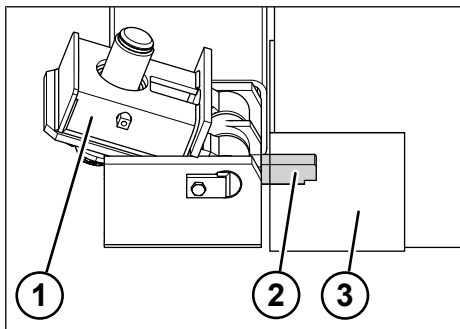
Fig. 6-21: Meccanismo di presa container in posizione di riposo
