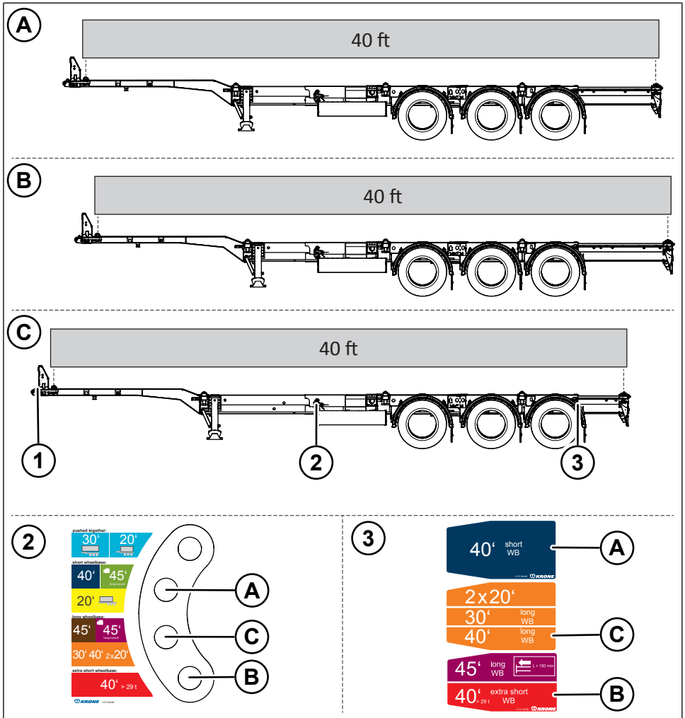
Fig. 6-29: Vista generale delle posizioni dei container
