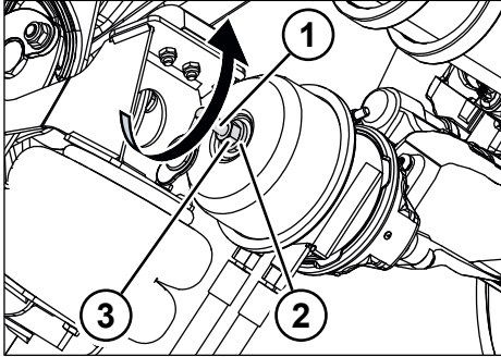
Fig. 5-15: Disattivare la vite per il rilascio di emergenza
