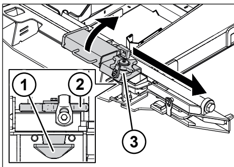
Fig. 6-15: Meccanismo di presa container in posizione di riposo
