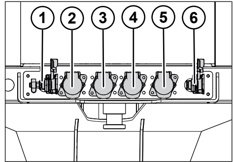
Fig. 5-6: Attacchi di alimentazione e comando
