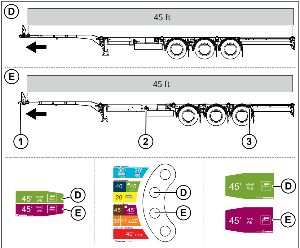
Fig. 6-31: Vista generale delle posizioni dei container
