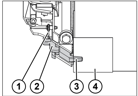
Fig. 6-19: Meccanismo di presa container in posizione di riposo
