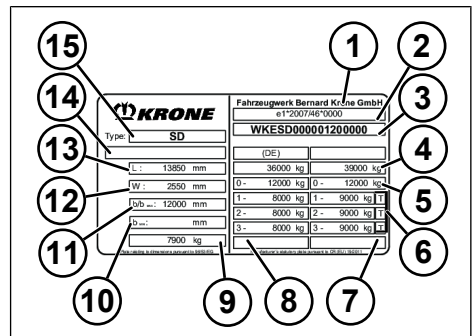
Fig. 1-1: Esempio di targhetta di fabbricazione
