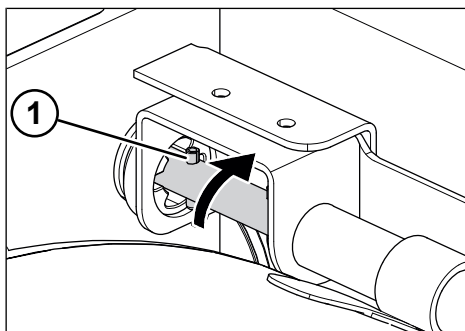
Fig. 6-7: Rotazione della manovella per allungamento posteriore
