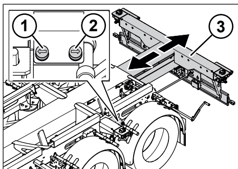
Fig. 6-11: Estrazione pneumatica dell'allungamento posteriore
