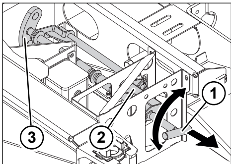
Fig. 6-2: Funzionamento allungamento centrale
