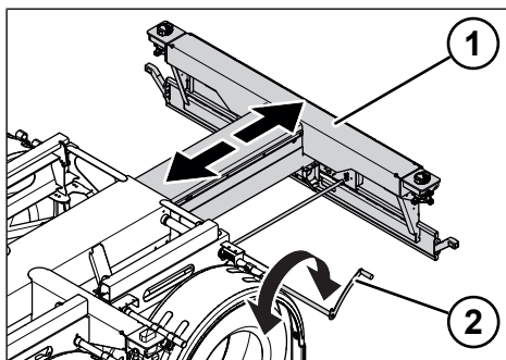
Fig. 6-6: Estrazione allungamento posteriore
