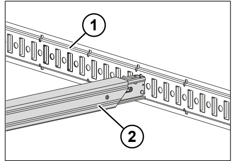
Fig. 8-10: Barre di bloccaggio
