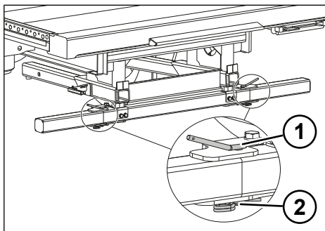
Fig. 5-27: Barra paraincastro orientabile su entrambi i lati
