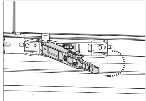
Fig. 6-3: Rotazione della leva per la chiusura porte
