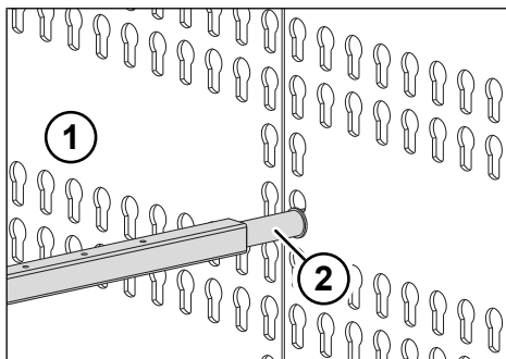
Fig. 8-11: Barra di bloccaggio lamiera a nido d'ape
