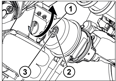
Fig. 5-17: Disattivare la vite per il rilascio di emergenza
