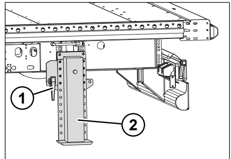
Fig. 5-8: Supporto posteriore ribaltato verso il basso
