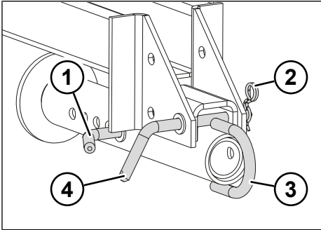
Fig. 5-9: Ribaltare verso il basso il supporto posteriore
