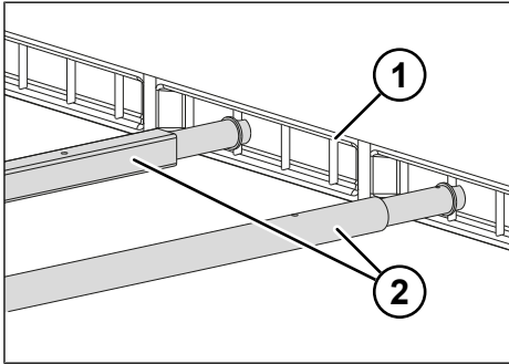
Fig. 8-9: Barre di fermo guida per barra fermacarico
