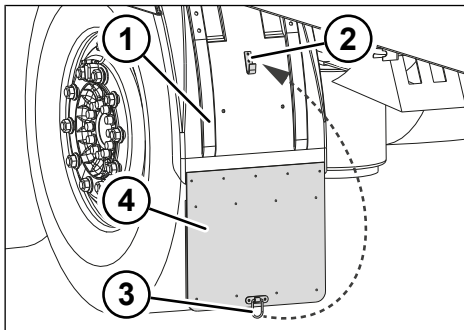
Fig. 5-32: Paraspruzzi ribaltati verso il basso
