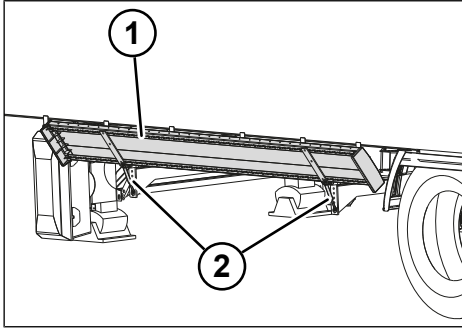
Fig. 5-29: Dispositivo di protezione laterale sollevato
