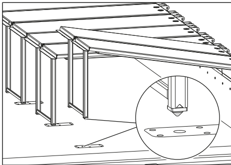
Fig. 6-24: Aiuto per posizionamento piede di appoggio
