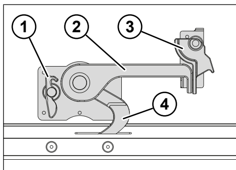
Fig. 6-14: Bloccaggio a gancio
