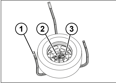
Fig. 5-33: Ruota di scorta con cestello di supporto, modello 1
