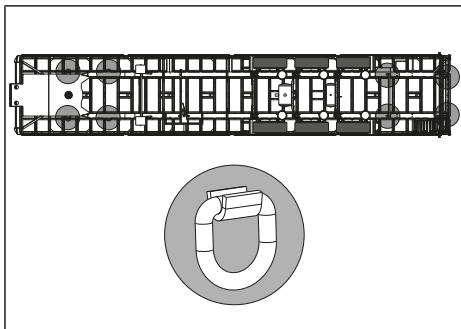
Fig. 7-4: Disposizione dei ganci nave
