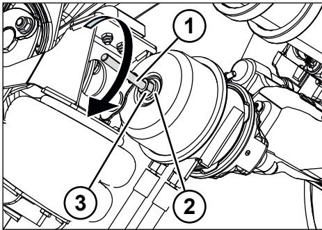
Fig. 5-16: Attivare la vite per il rilascio d'emergenza
