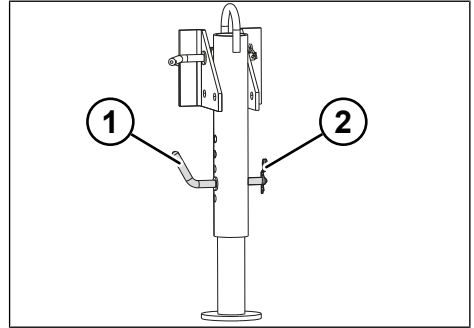
Fig. 5-10: Regolare l'altezza del supporto posteriore
