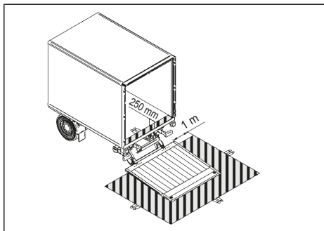
Fig. 6-11: Area di pericolo della sponda montacarichi
