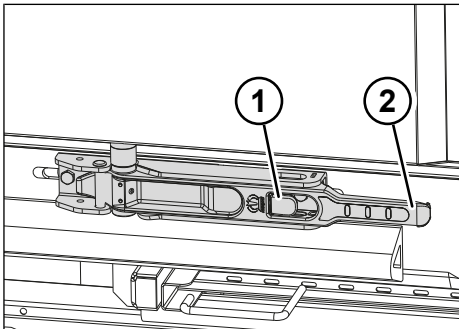
Fig. 6-2: Chiusura delle porte con azionamento a una mano
