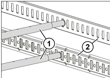
Fig. 8-8: Barre di fermo guida fermacarico combinata
