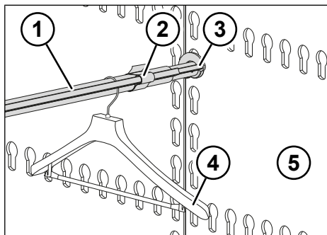
Fig. 8-12: Barre per indumenti
