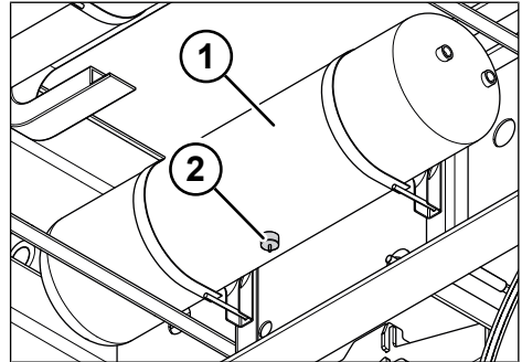
Fig. 5-14: Serbatoio dell'aria compressa
