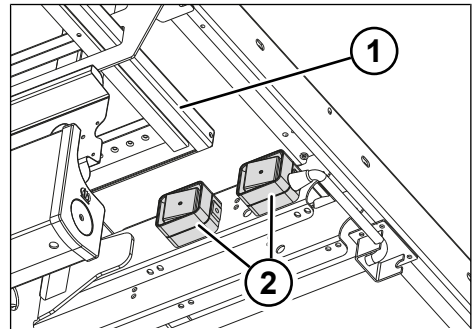
Fig. 6-18: Interruttore sul telaio
