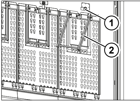
Fig. 6-23: Sganciare il piede di appoggio
