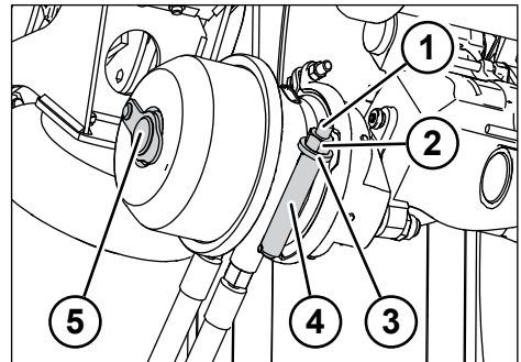
Fig. 5-15: Accumulatore a molla con dispositivo di rilascio di emergenza
