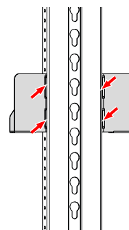
Kapsy profilu na středním sloupku (svařované nebo nýťované)
