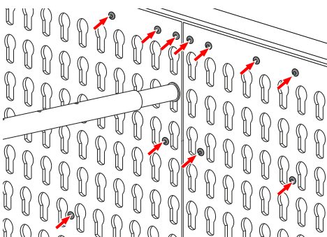
Plech s otvory ve tvaru klíčových dírek nahoře
