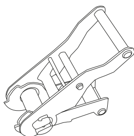
Ráčna (zajištění přes úvrat')
