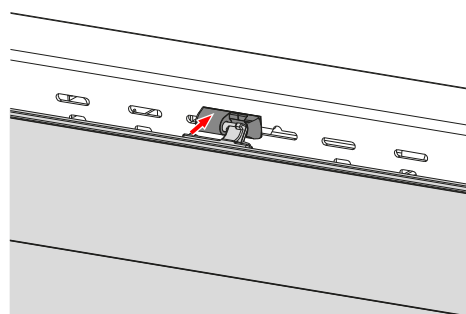
Ložisko pantu na podlahovém rámu
