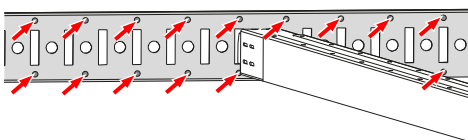
Kolejnice pro zajištění nákladu
