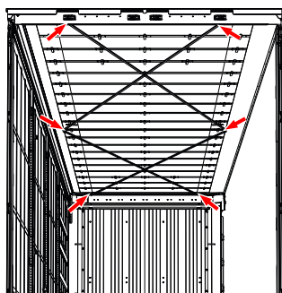
Diagonální popruhy (napnutí, všechny upevňovací body)
