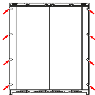
Dveřní závěsy – vnitřní tyčové uzávěry
