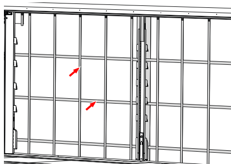
Plachta a vnitřní zesílení plachty (vertikální a horizontální)
