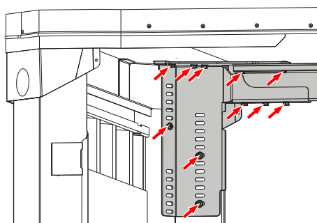
Střešní oblouk a přední rohový sloupek
