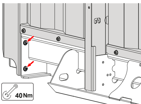
Přední rohový sloupek (plachtová nástavba)
