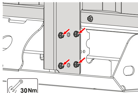
Podpěra čelní stěny
