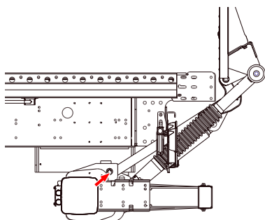
Vertikální zvedací nakládací plošina
