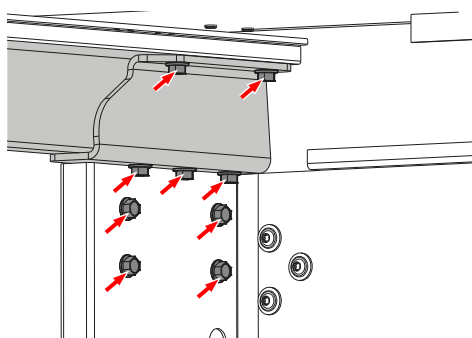
Střešní oblouk a zadní rohový sloupek
