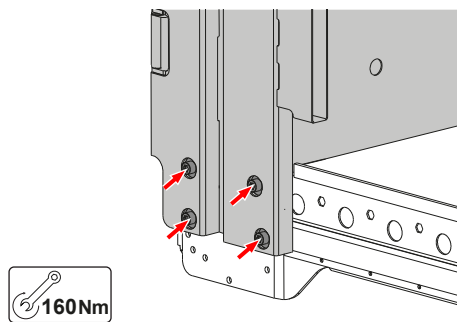
Zadní rohový sloupek (plachtová nástavba)
