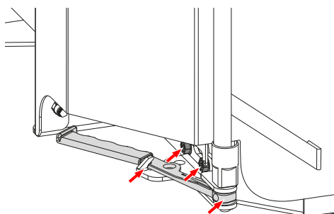
Přední napínací páka (šroubový spoj, ráčna a uvolňovací mechanismus)
