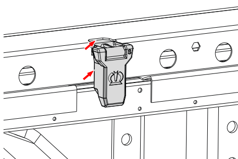
Uložení středového sloupku na podlahovém rámu (svařované)
