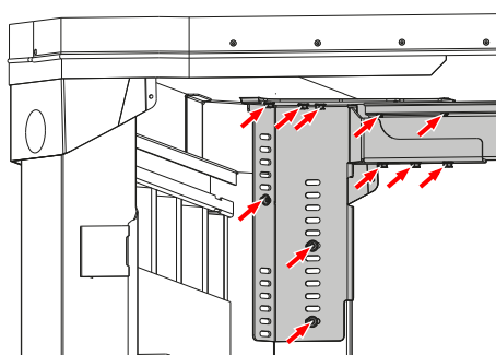
Tagstiver og hjørnestolpe foran
