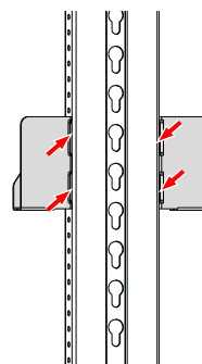
Bræddeholdere på midterstolpe (svejset eller nit-tet)
