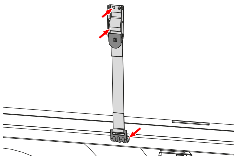
Presenningspændere (antal) og spændekroge (krogospænding)
