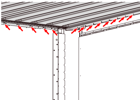
Tag (indvendigt)
