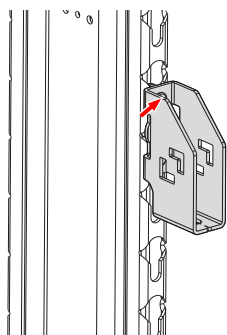
Bræddeholder til dobbeltdæk i hjørnestolpe og midterstolpe (strakt)
