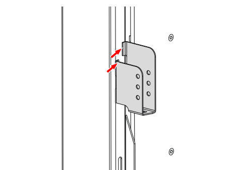
Bræddeholdere på hjørnestolper – forvæg og bagportal (svejet eller skruet)
