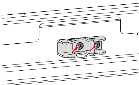
Modholder øverst – indvendige lukkestænger
