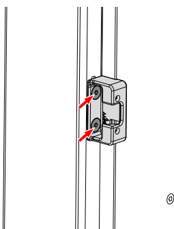
Modholder på hjørnestolper og midterstolper
