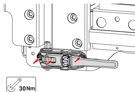
Spændeskralde bagved (forskruning og skralde)
