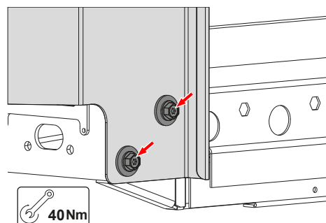
Hjørnestolpe i siden (presenningkarosseri)
