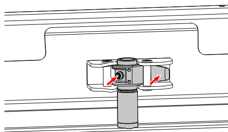
Dørlås øverst – indvendige lukkestænger (krogopspænding)
