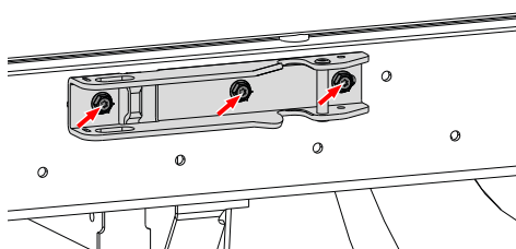
Modholder nederst – indvendige lukkestænger
