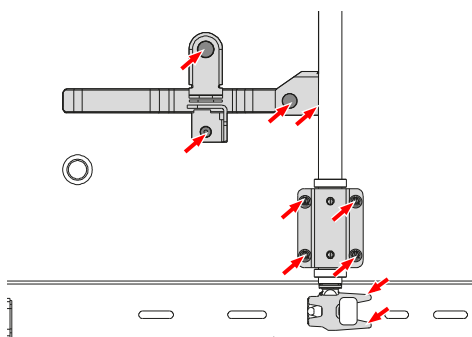
Dørlås nederst – udvendige lukkestænger
