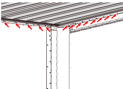
Tak (innvendig)
