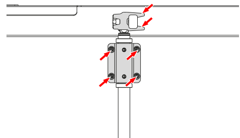
Dørlås oppe - utvendige dreiestenger (krokoppspenning)
