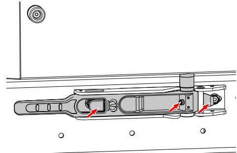
Dørlås nede - innvendige dreiestenger (krokoppspenning)
