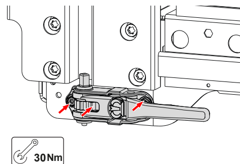
Strammeskralle bak (skrueforbindelse og skralle)
