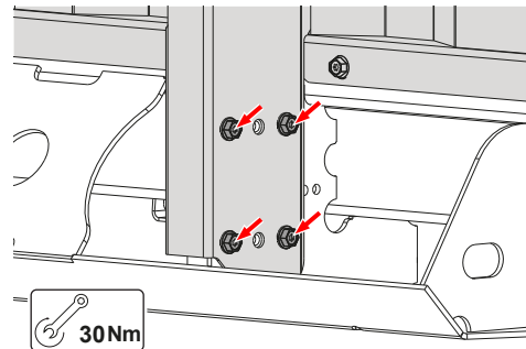
Frontveggstøtte
