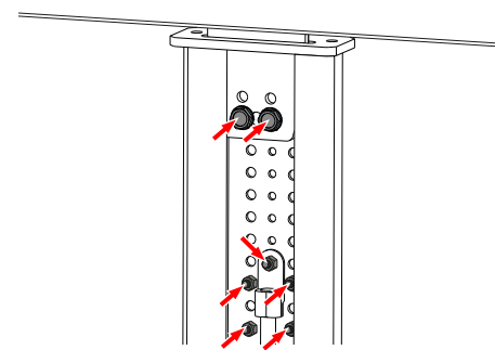
Midtstolpe oppe
