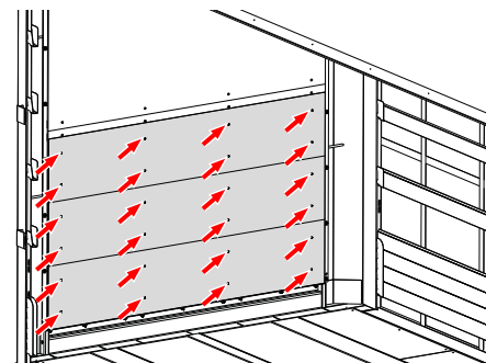
Støtbeskyttelsesplate innvendig
