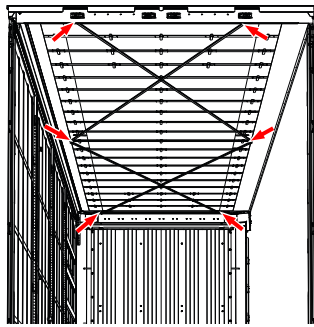
Diagonalstropper (stramming, alle festepunkter)
