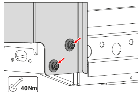
Hjørnestolpe på siden (presenningpåbygg)
