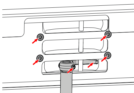
Dørlås oppe – hevetak (krokoppspenning)
