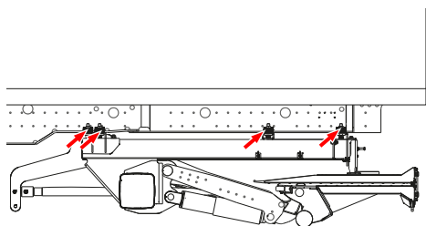
Stående heveplattform
