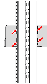
Sprosselomme midtstolpe (sveiset eller naglet)
