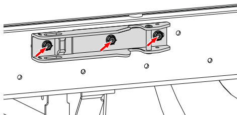
Motholder nede - innvendige dreiestenger
