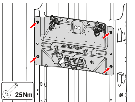
Koblingsholdere
