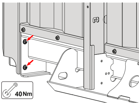
Hjørnestolpe foran (presenningpåbygg)
