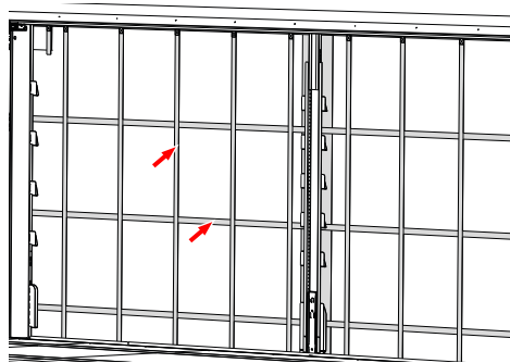
Presenning og innvendig presenningforsterkning (vertikal og horisontal)
