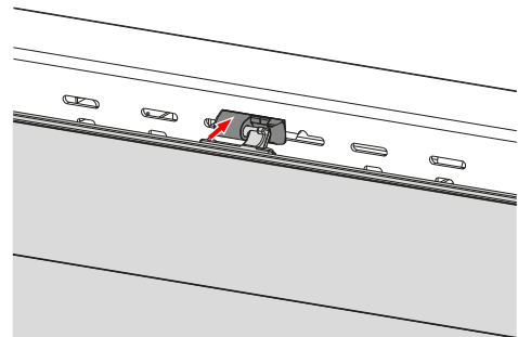
Hengsellager på bunnrammen
