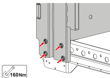
Hjørnestolpe på bakenden (presenningpåbygg)
