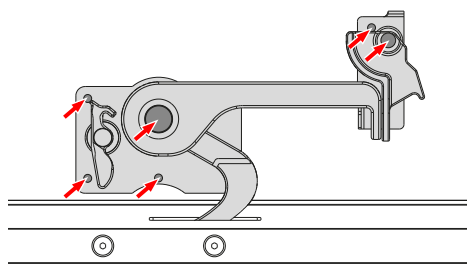
Rulledørlås
