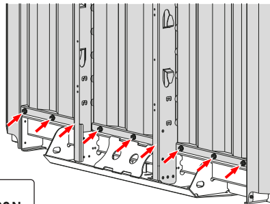
Frontvegg foran
