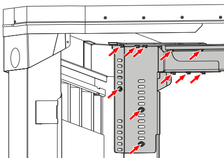
Takbøyle hjørnestolpe foran
