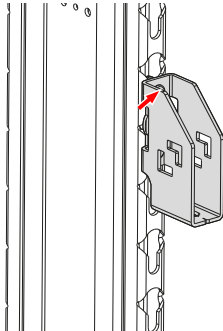
Sprosselomme dobbeletasjestolpe i hjørnestolpe og midtstolpe (strukket)
