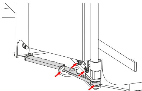
Strammespak foran (skrueforbindelse, skralle og løseanordning)
