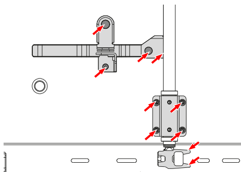
Dørlås nede - utvendige dreiestenger
