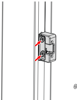
Motholdere på hjørnestolper og midstolper
