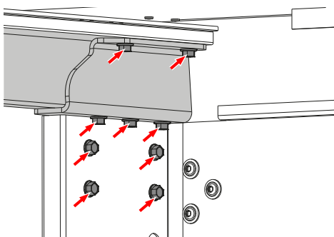
Takbøyle og hjørnestolpe bak
