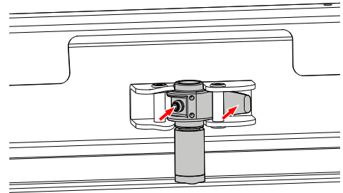
Dørlås oppe - innvendige dreiestenger (krokoppspenning)
