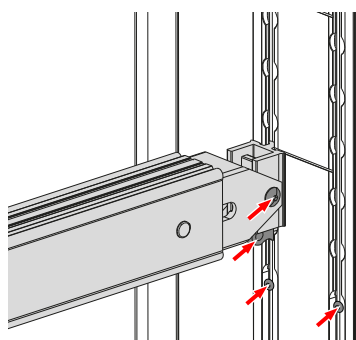
Dobbeletasje-bæreelement og skinne
