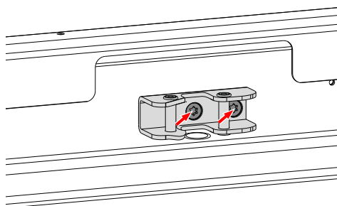
Zgornje protidrżalo – notranji vrtljivi drogovi
