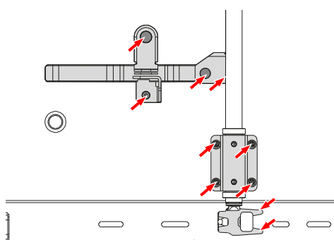
Spodnja ključavnica vrat – zunanji vrtljivi drogovi
