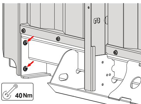
Sprednja kotna ročica (nadgradnja s ponjavo)
