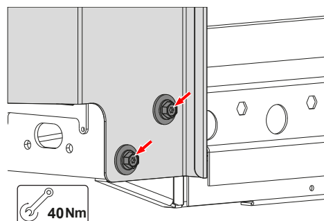
Stranska kotna ročica (nadgradnja s ponjavo)
