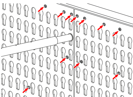
Pločevina z luknjo za ključ zgoraj
