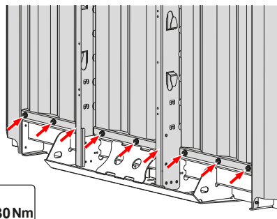
Sprednja čelna stena
