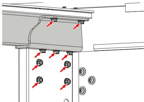
Strešni loki in kotna ročica zadaj
