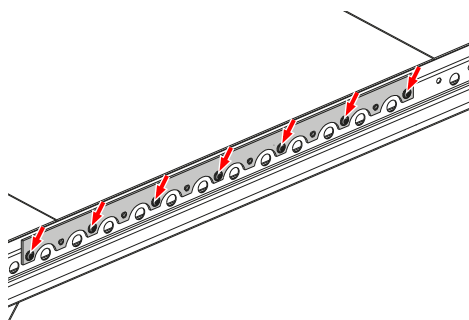
Nastavki za privezovanje palet (priviti ali varjeni)
