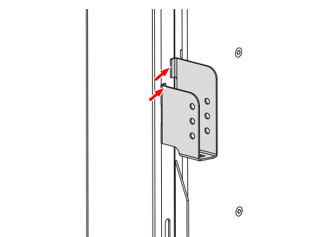
Vložno mesto za letve na kotnih ročicah – čelna stena in zadnja odprtina (varjeno ali privito)
