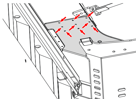
Notranji strešni pokrov
