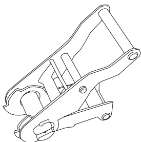
Zatič (varovalo prek mrtve točke)
