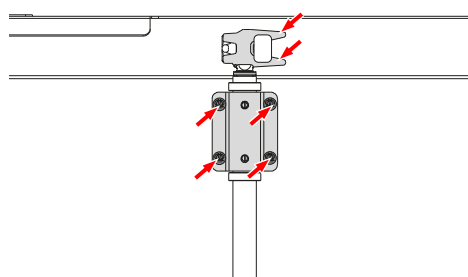
Zgornja ključavnica vrat – zunanji vrtljivi drogovi (vpenjanje s kavlji)
