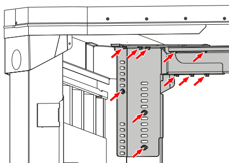
Strešni loki in kotna ročica spredaj
