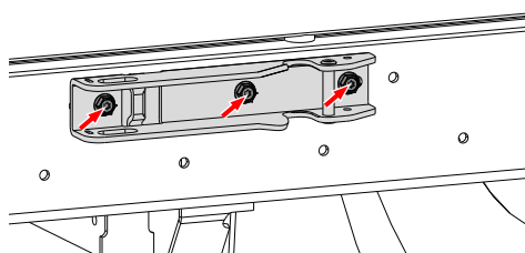
Spodnje protidrżalo – notranji vrtljivi drogovi
