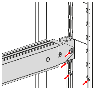
Dvonadstropni nosilni element in tirnica
