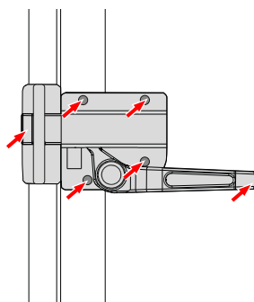
Zaklepanje stoječega drsnega nakladalnega odra
