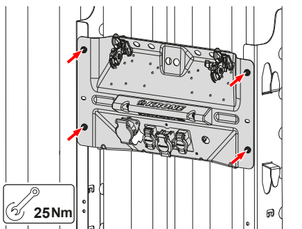
Nosilec spojke
